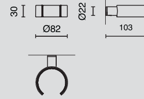
Föhnhalter / hair drier holder NR. 40241
