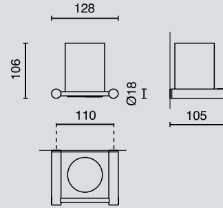
Zahnputzglas / tumbler, NR. 40266
