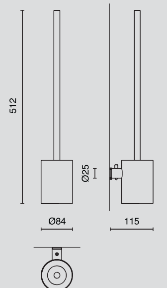
Toilettenbürste * / toilet brush *, NR. 40255
