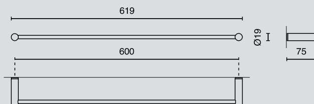
Handtuchstange / towel rail, NR. 40252
