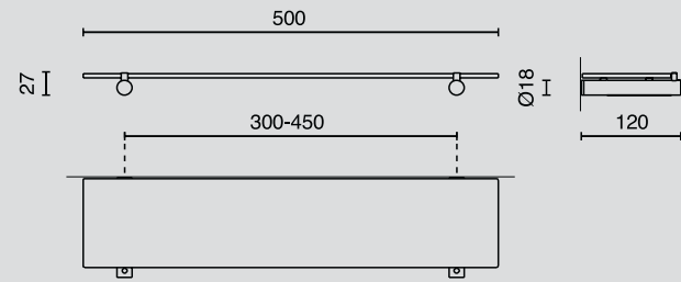
Glasablage / bathroom shelf, NR. 40256
