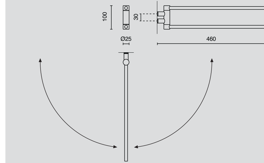
Handtuchstange / towel rail, NR. 40246
