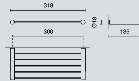
Handtuchablage / towel shelf, NR. 40258
