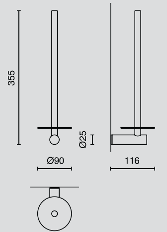
Ersatzrollenhalter / spare toilet roll holder, NR. 40261
