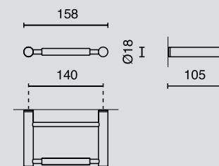
Toilettenpapierhalter / toilet roll holder, NR. 40254
