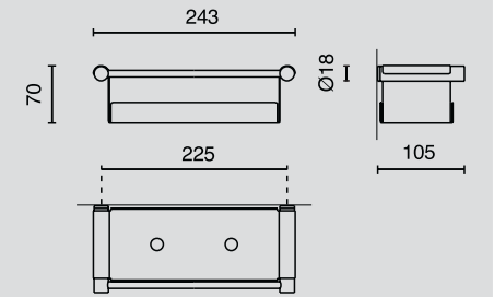
Utensilienkorb / bathroom basket, NR. 40257
