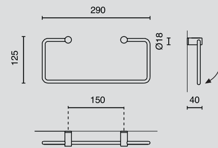
Handtuchring / towel holder, NR. 40260
