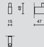
Handtuchhaken / towel hook NR. 40390
