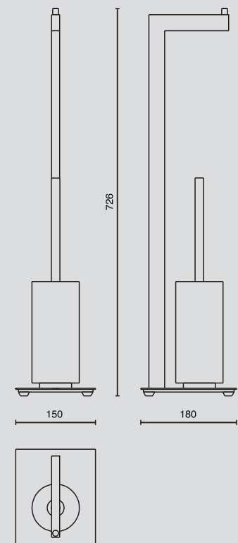
Toilettenbutler * / toilet butler *, H. 72,5 cm NR. 40382
